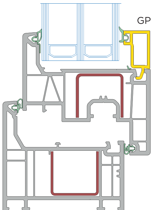
Trojsklo, zasklievacia lišta rovná
