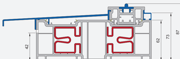
HSB 176 + HSB 276 s vypusteným prekrytím
