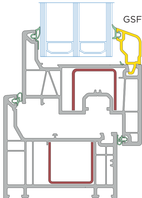
Trojsklo, zasklievacia lišta zaoblená
