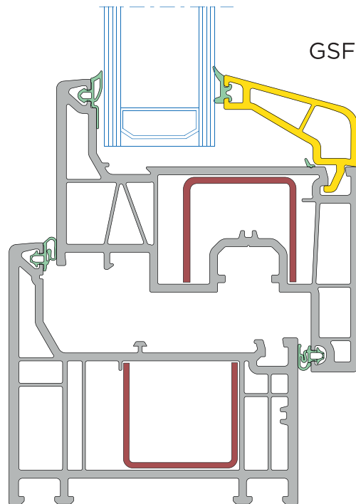
Dvojsklo, zasklievacia lišta zaoblená
