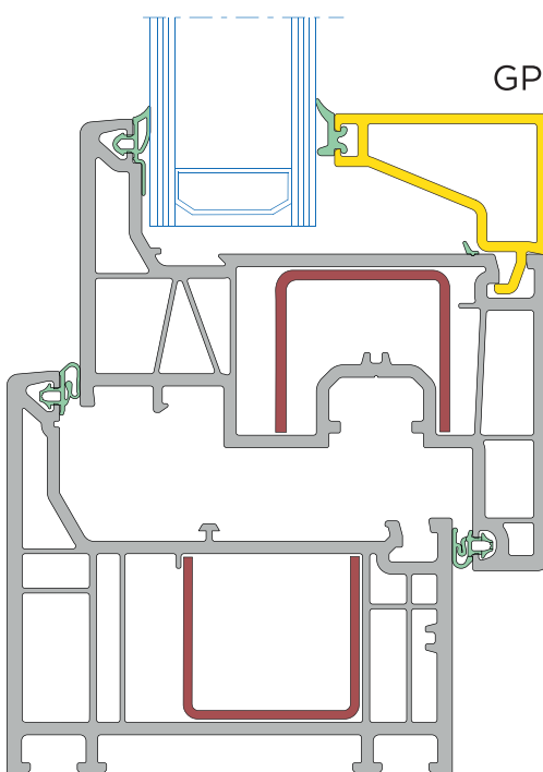
Dvojsklo, zasklievacia lišta rovná
